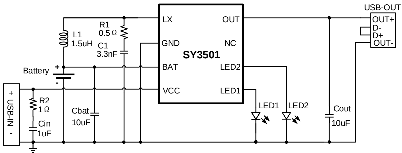
SY3501 典型应用电路
